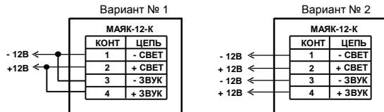
Рис.1 Схема подключения.
