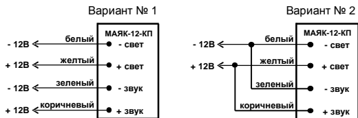
Рис.1 Схема подключения.
