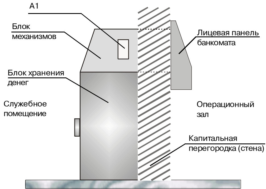
Рисунок В.7 - Установка извещателя (ДВ) на банкомате, встроенном в капитальную строительную конструкцию
