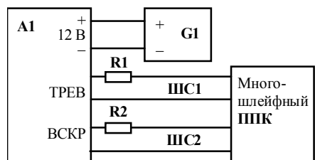
Схема подключения извещателя "Шорох-2" с отдельной передачей извещений "Тревога" и "Вскрытие"
